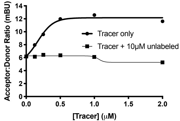
NL-DSTYK Tracer 10-7600 Staurosporine EC50
